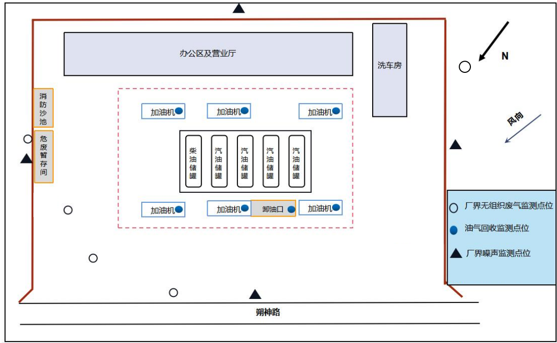
图 3-1 中国石化销售股份有限公司山西朔州建设北路加油站监测点位布设图 (注：以实际监测时气象条件为准)
