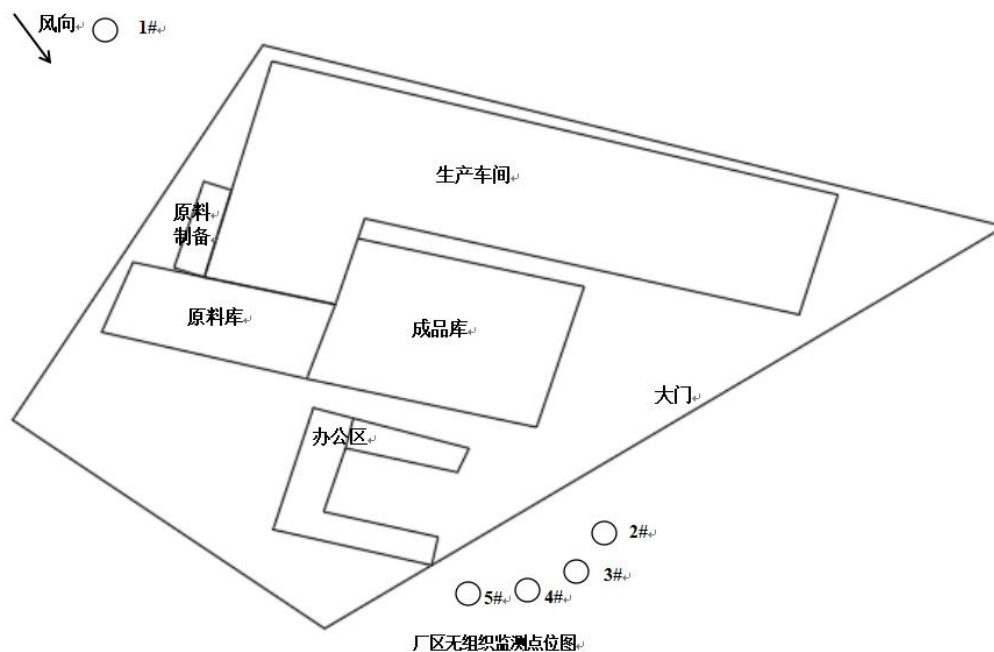
图 3-3 厂界无组织监测点位示意图
