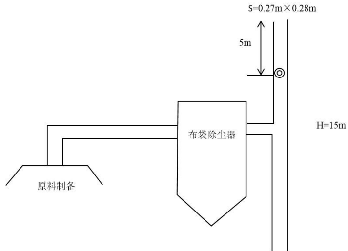
图3-2 2#原料破碎废气排放口监测点位示意图
