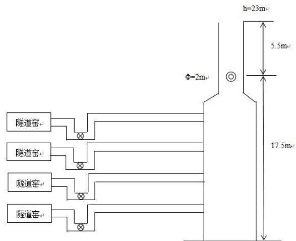
图3-4 隧道窑废气总排放口监测点位示意图
