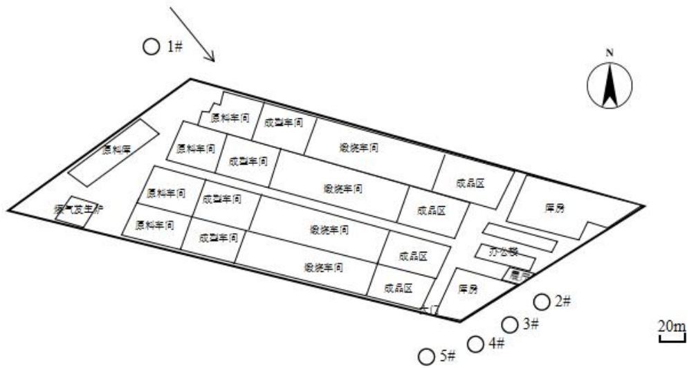
图3-5 厂界无组织监测点位示意图
