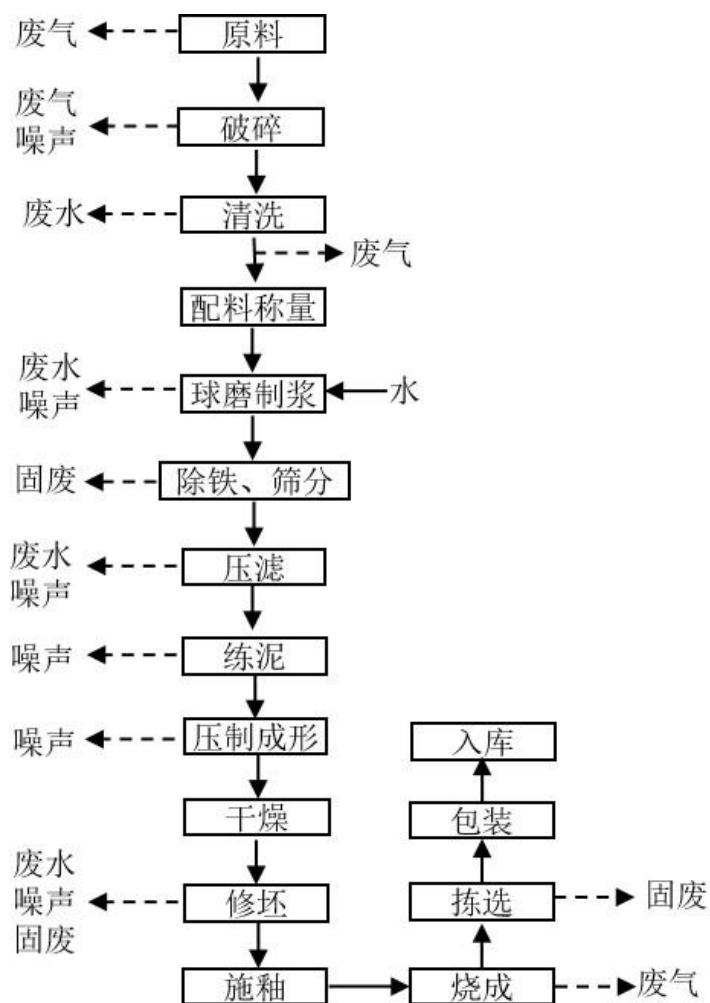
图1-1 本项目工艺流程图
