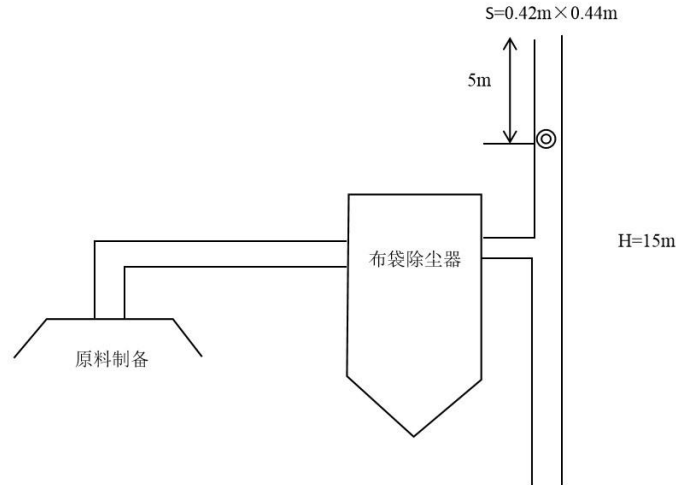
图3-1 1#原料破碎废气排放口监测点位示意图
