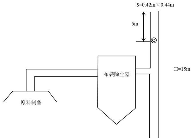
图3-3 3#原料干碾废气排放口监测点位示意图
