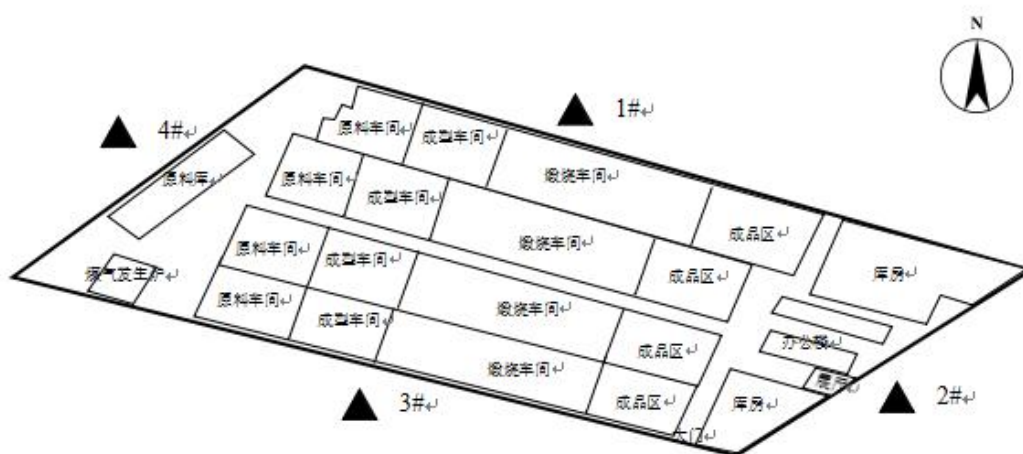
图 3-6 厂界噪声监测点位示意图
