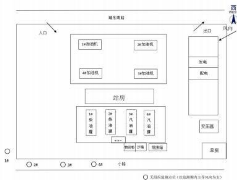
图 3-1 厂界无组织废气手工监测点位示意图 (以监测期间主导风向为主)
