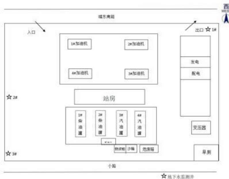
图 3-3 地下水手工监测点位示意图
