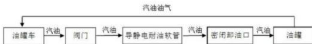
汽油卸油工艺
