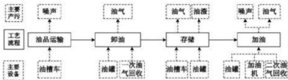
产物环节及治理设施
