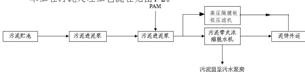
图1-2 污泥处理工艺流程图
