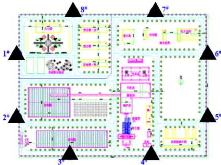
图 3-13 厂界噪声监测布点示意图
