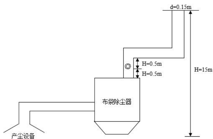
图3-1 1#布袋除尘器废气排放口、2#布袋除尘器废气排放口、3#布袋除尘器废气排放口监测点位示意图
