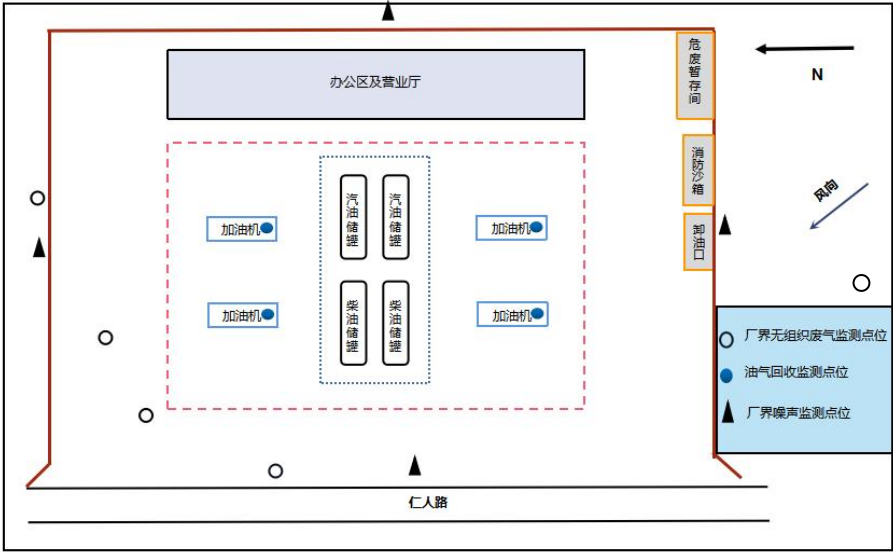
图 3-1 中国石化销售股份有限公司山西朔州怀仁怀同路加油站监测点位布设图
