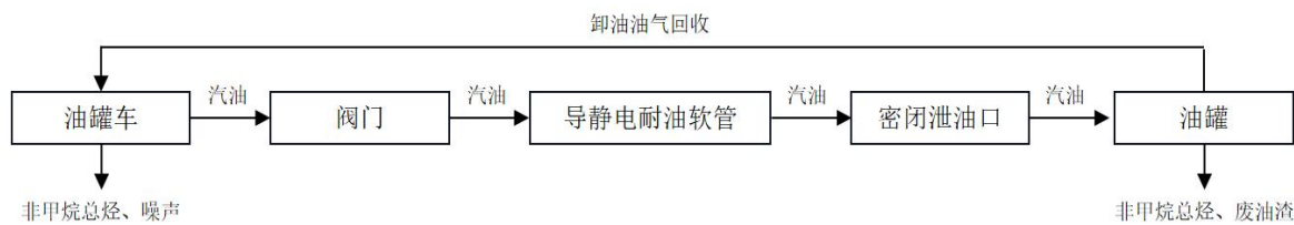
图 1-1 汽油卸油与产污工艺流程图
