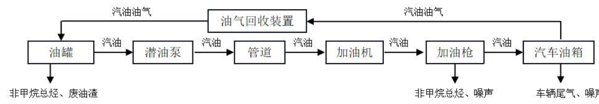
图 1-2 汽油加油与产污工艺流程图
