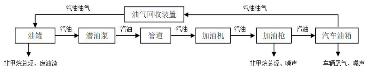
图 1-1 卸油、加油、油气回收工艺流程图
