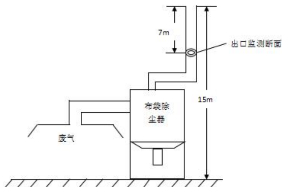
图 3-4 四期工程破碎工序布袋除尘器监测点位图
