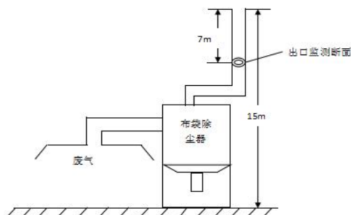
图 3-1 一期工程破碎工序布袋除尘器监测点位图
