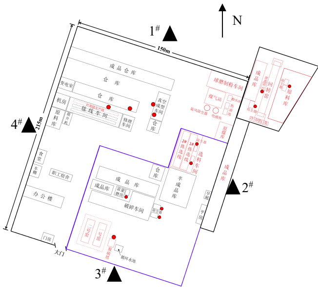
图 3-7 厂界噪声监测点位示意图
