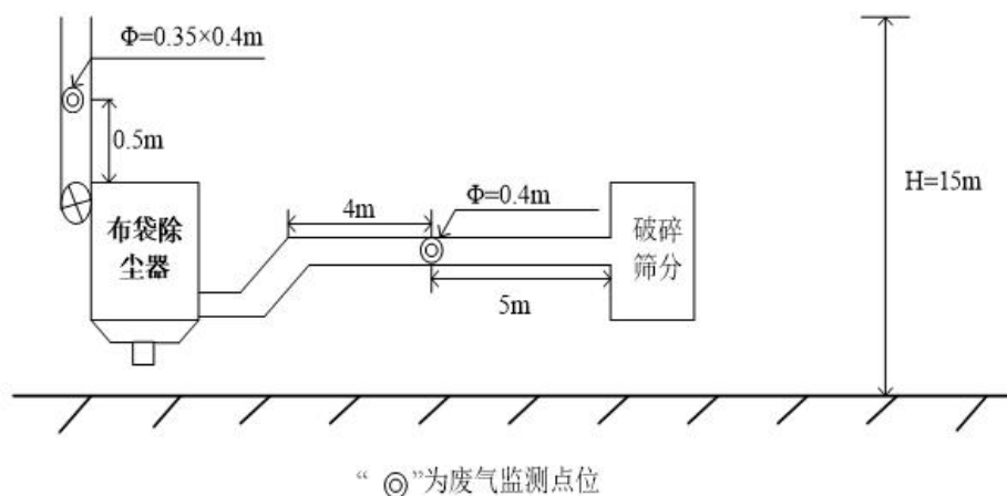
图3-4 2#破碎筛分废气排放口监测点位示意图
