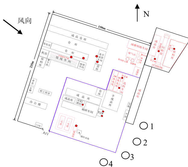
图3-5 粉磨废气排放口监测点位示意图
