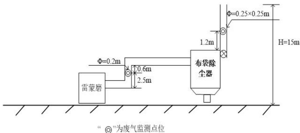
图3-5 粉磨废气排放口监测点位示意图
