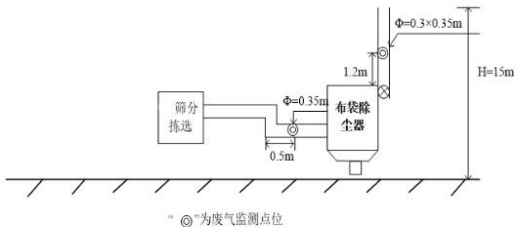
图 3-1 筛分拣选废气排放口监测点位示意图
