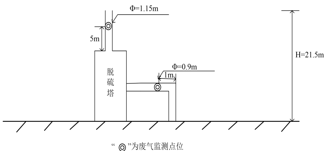
图 3-2 环式节能密封烟气排放口监测点位示意图
