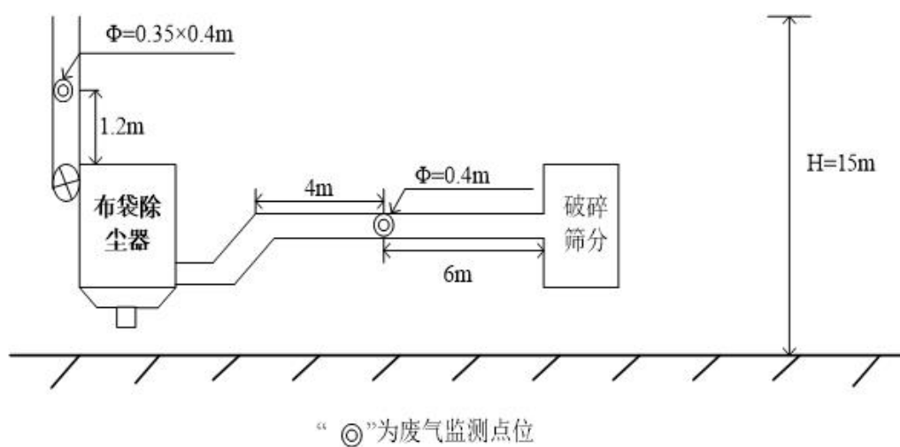
图 3-3 1#破碎筛分废气排放口监测点位示意图
