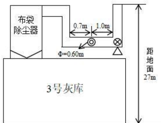
3号灰库顶部除尘器监测点位示意图
