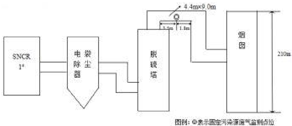
锅炉固定污染源废气监测点位示意图
