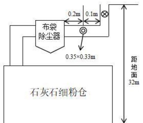
石灰石细粉仓布袋除尘器监测点位示意图
