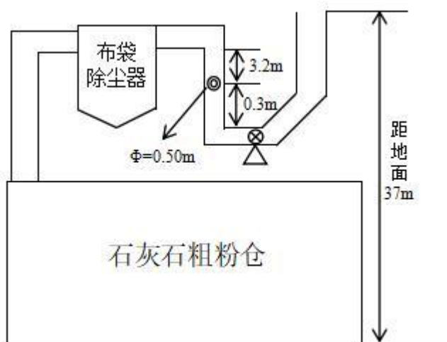
石灰石原料仓布袋除尘器监测点位示意图
