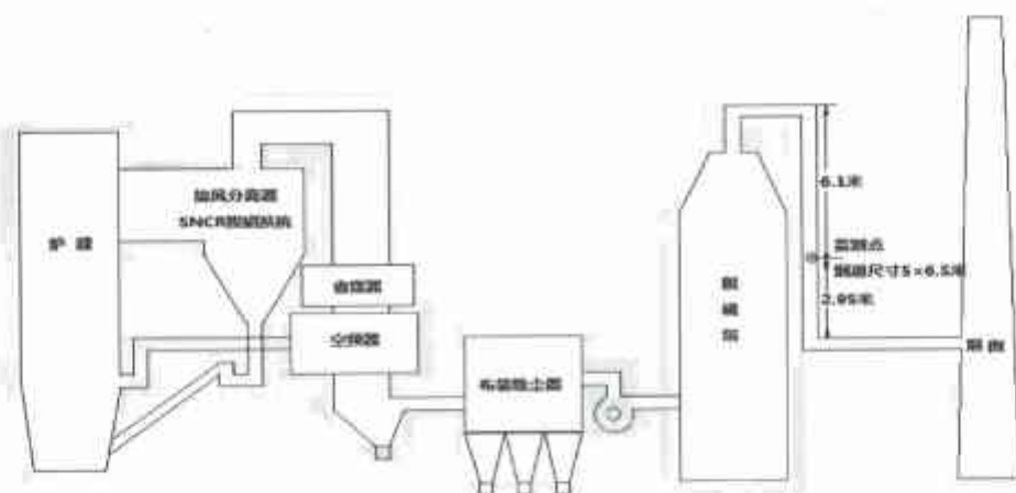
图 3-1 3、4 机组锅炉脱硫塔后烟道固定污染源废气监测点位示意图
