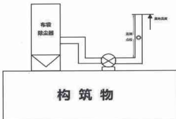
图 3-4 一般排放口固定污染源废气监测点位示意图
