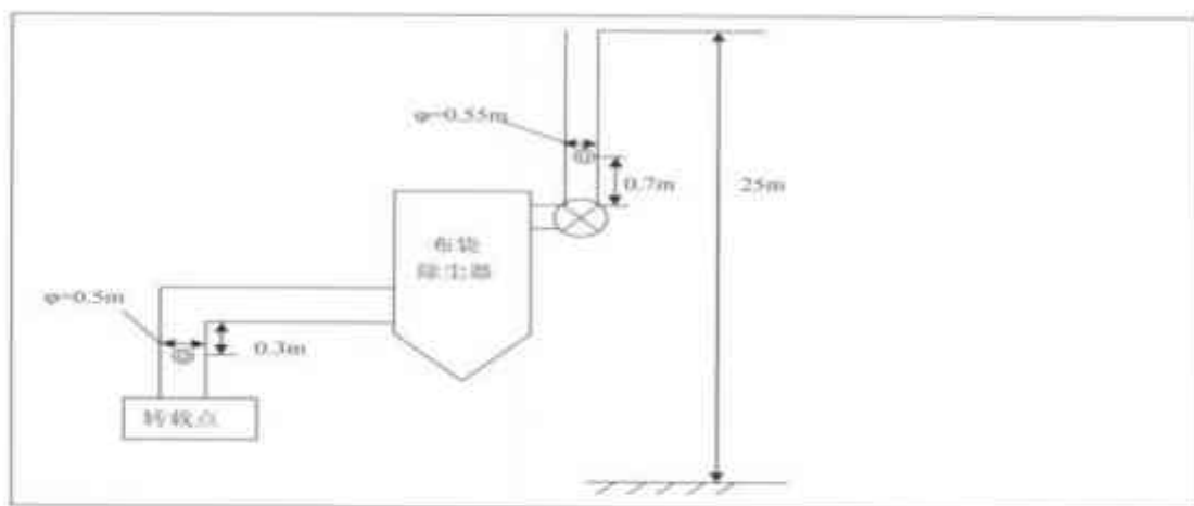
图 3-2 1#转运站 1#、2#布袋除尘器监测点位示意图
