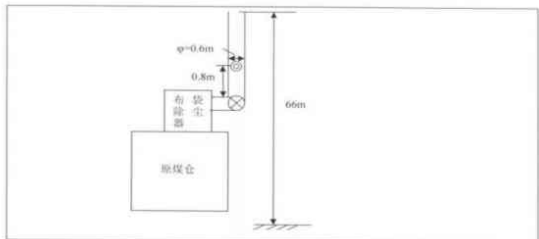
图 3-4 #1-#8 原煤仓布袋除尘器监测点位示意图
