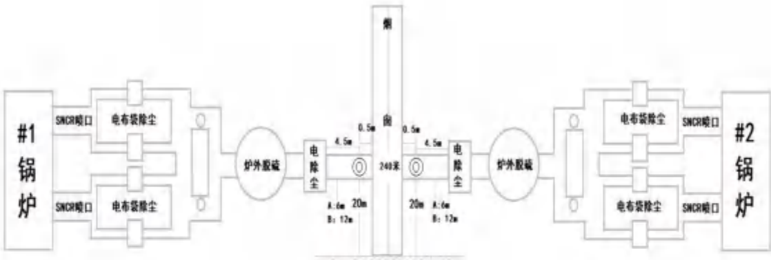
锅炉烟气手工监测点示意图
