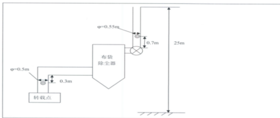
图 3-2 1#转运站 1#、2#布袋除尘器监测点位示意图
