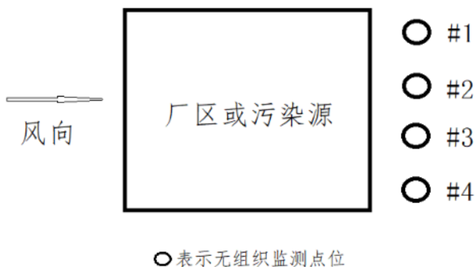
图 3-8 厂界无组织废气监测点位示意图
