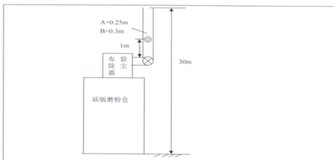
图 3-7 制粉车间欧版磨煤机布袋除尘器监测点位示意图
