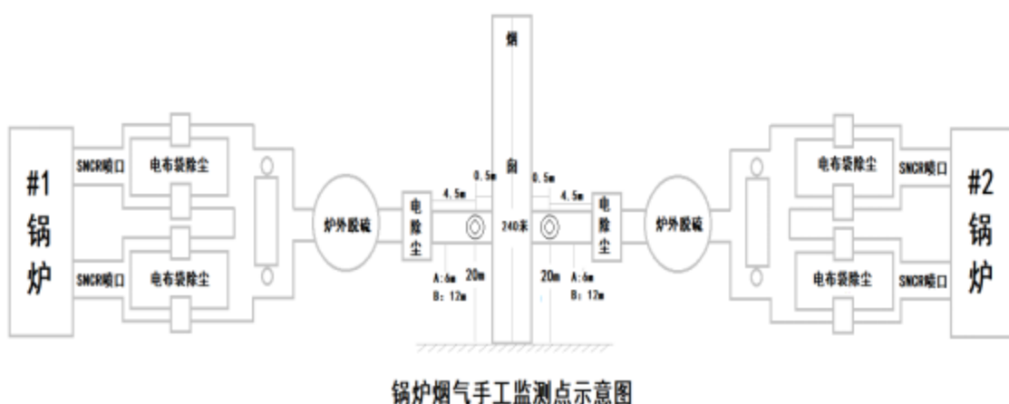
图 3-1 固定污染源汞及其化合物监测点位图
