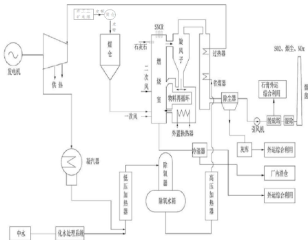
图 1-1 生产工艺流程图
