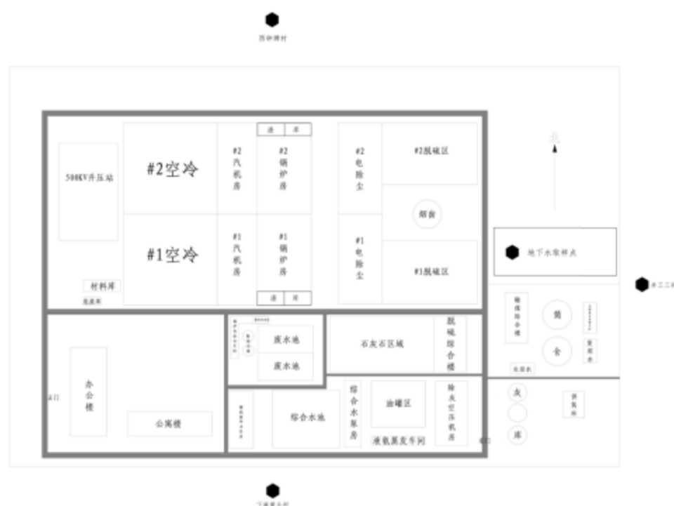
图 3-11 周边环境质量监测点位示意图
