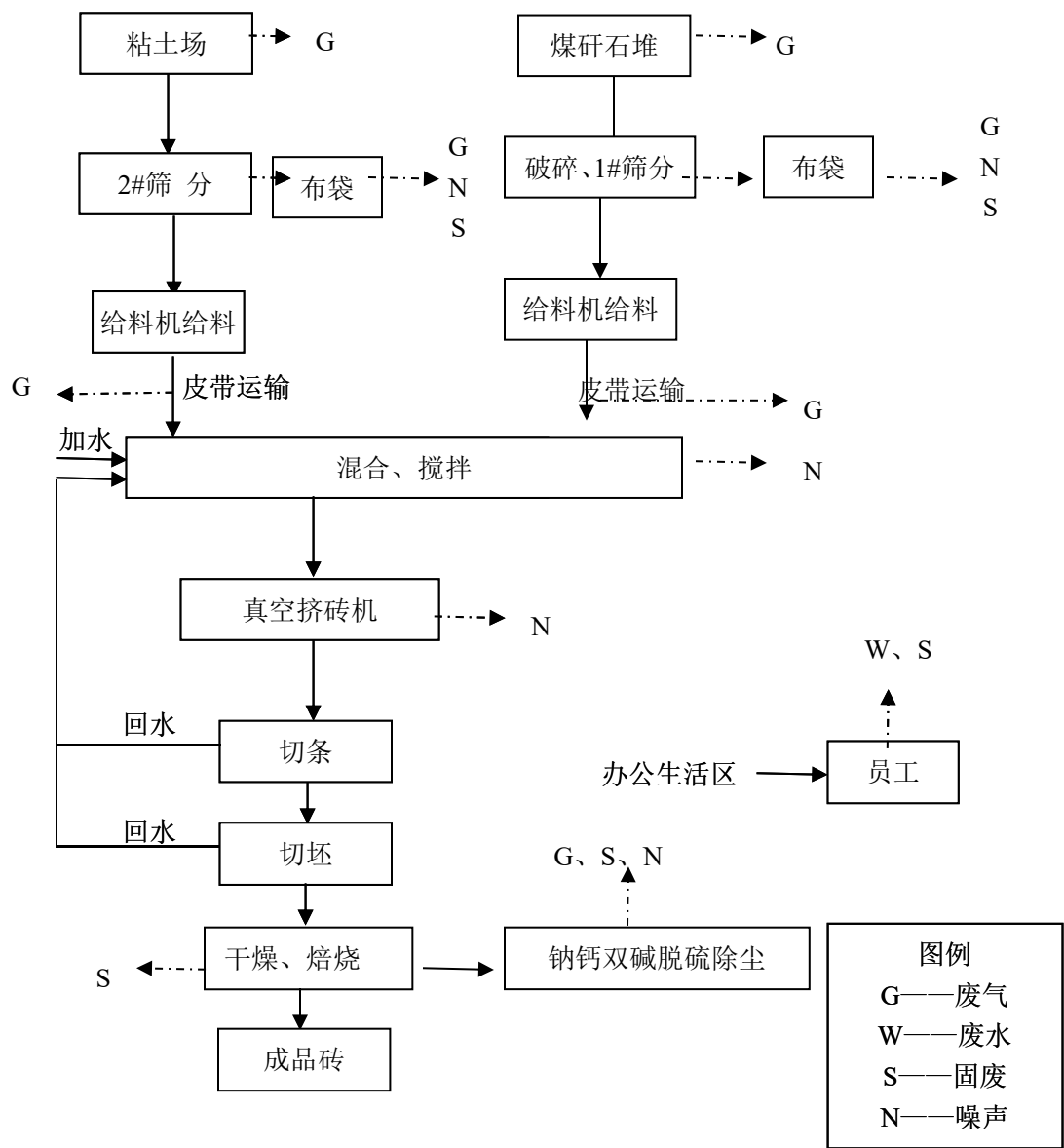
图 1-1 制砖生产工艺及产排污环节流程图
