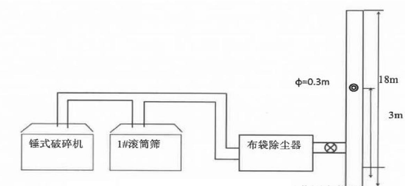
图 3-1 煤矸石锤破碎机和 1#滚筒筛废气排放口监测点位示意图（DA001）
