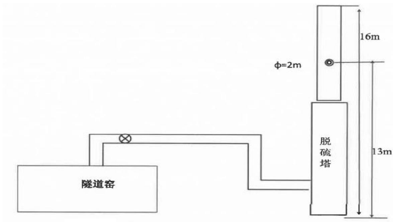
图 3-3 隧道窑废气监测布点示意图 (DA003)
