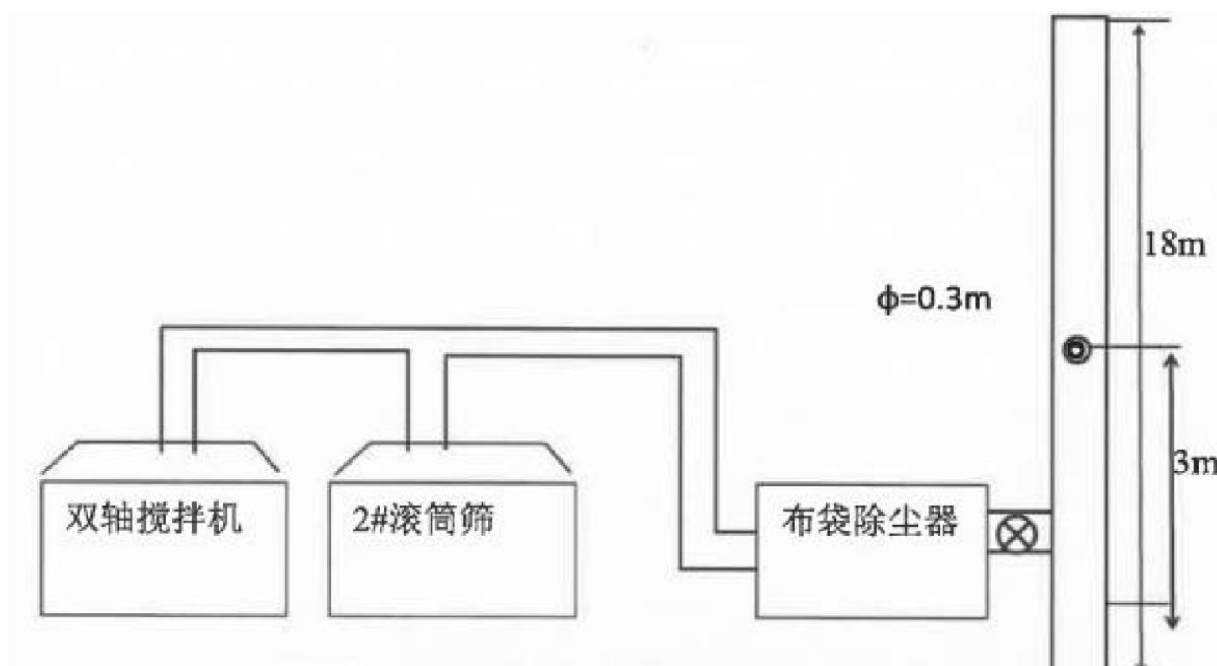
图 3-2 2#滚筒筛和双轴搅拌机废气排放口监测点位示意图 (DA002)
