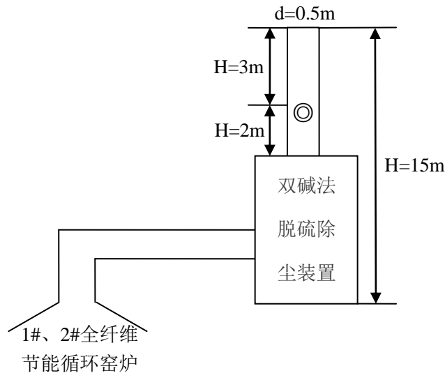
图 3-1 全纤维节能循环窑炉废气排放口监测点位示意图
