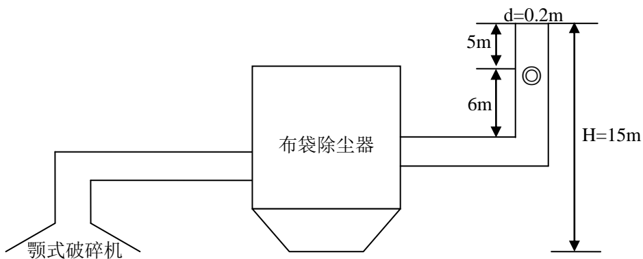
图3-2 破碎废气排放口监测点位示意图
