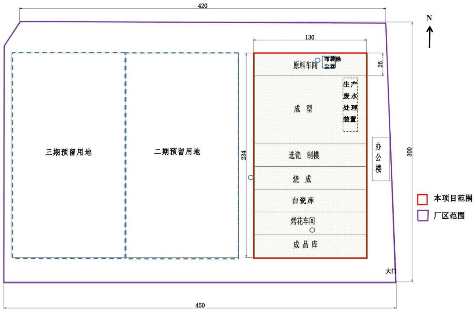
图 3-4 废水监测点位示意图
