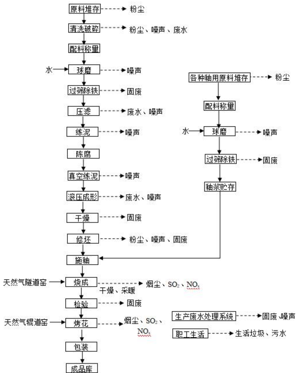
图 1-1 生产工艺流程图及产污节点
