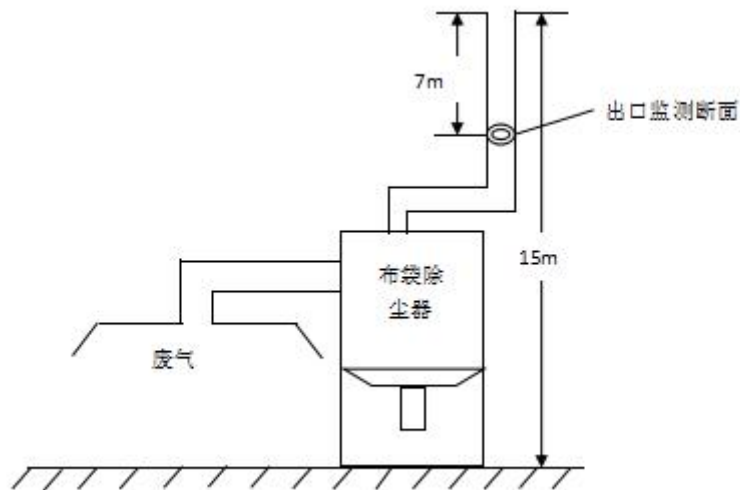
图 3-1 布袋除尘器监测点位图
