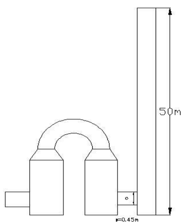
图3-6 灰锁泄压排气监测点位示意图
