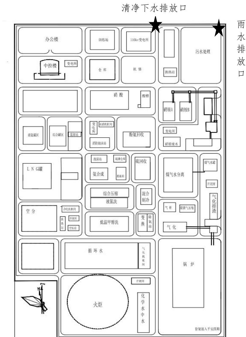
图 3-16 劣质煤项目生产区废水监测点位示意图
