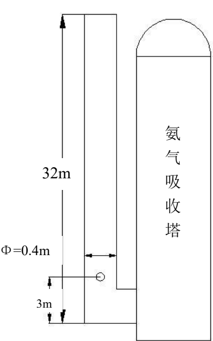
图3-13 氨气吸收塔排口监测点位示意图
