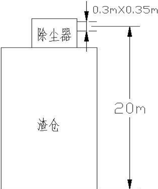
图3-11 渣库排口监测点位示意图
