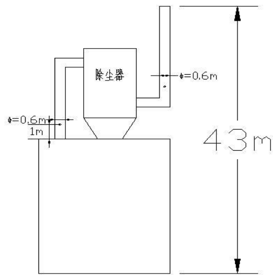
图3-3 原料气制备备煤筛分机排口监测点位示意图
