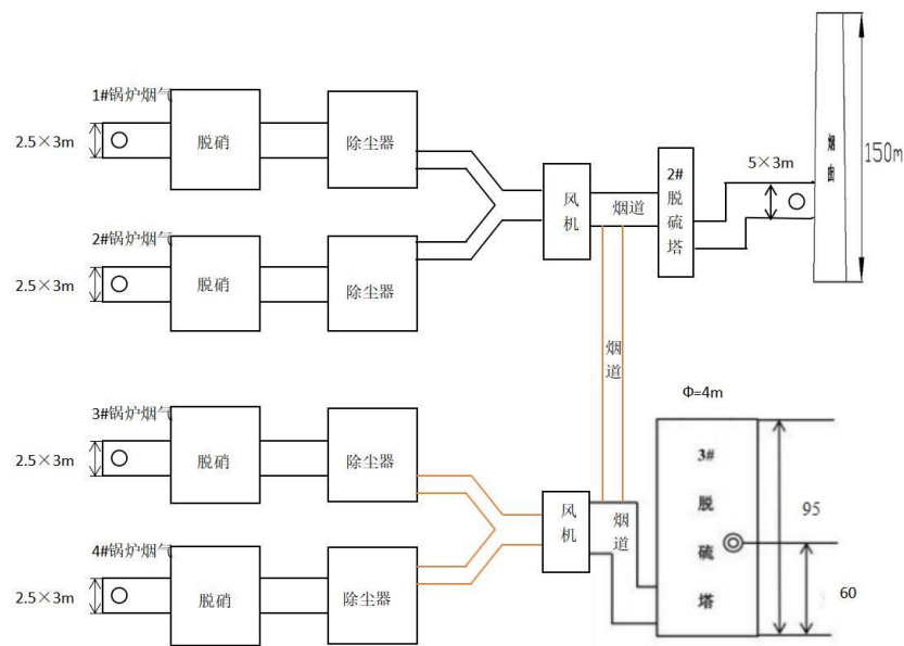
图3-1 动力锅炉脱硫塔出口监测点位示意图
