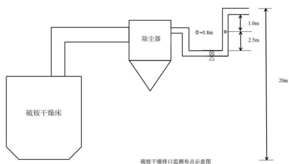
图3-5 硫铵干燥排口监测点位示意图
