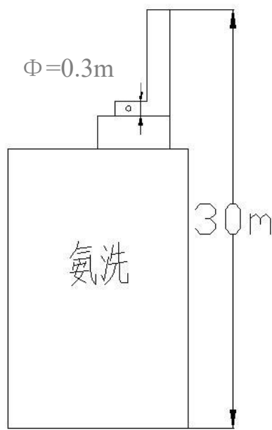
图3-1 动力锅炉脱硫塔出口监测点位示意图
