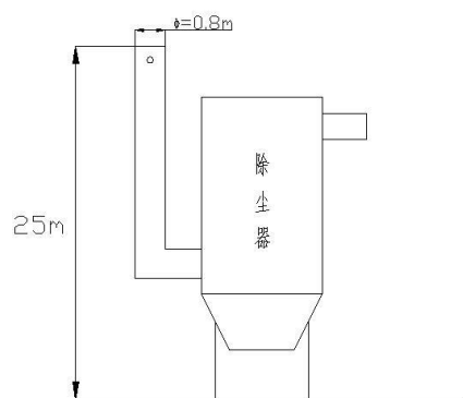
图3-4 硝铵包装机1#、2#排口监测点位示意图
