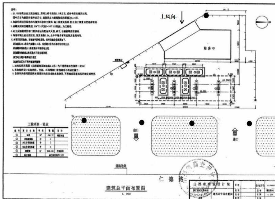
图 3-2 无组织废气监测点位示意图
