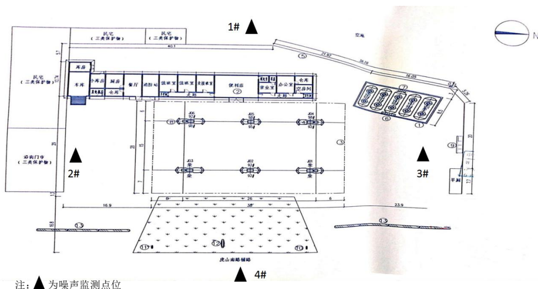
右玉油坊大桥加油站噪声监测示意图
