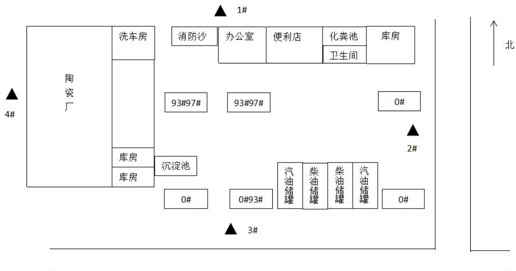
图 3-3 厂界噪声监测点位示意图
