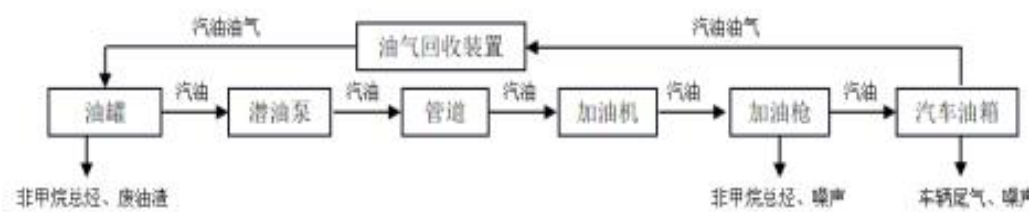
图 1-2 汽油加油与产污工艺流程图
