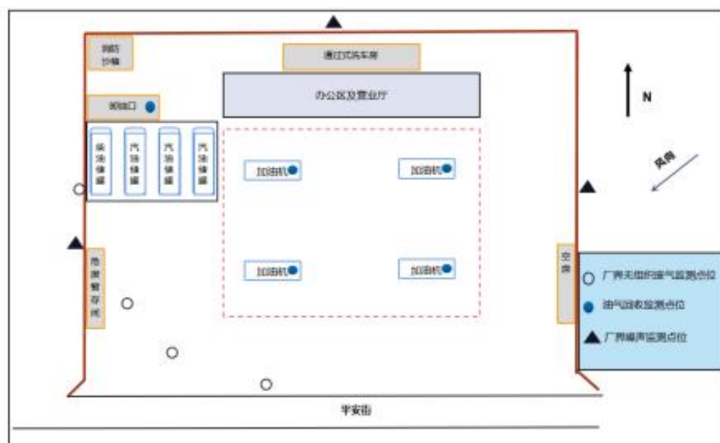
图 3-1 中国石化销售股份有限公司山西朔州平鲁平安东街加油站监测点位布设图 (注：以实际监测时气象条件为准)
