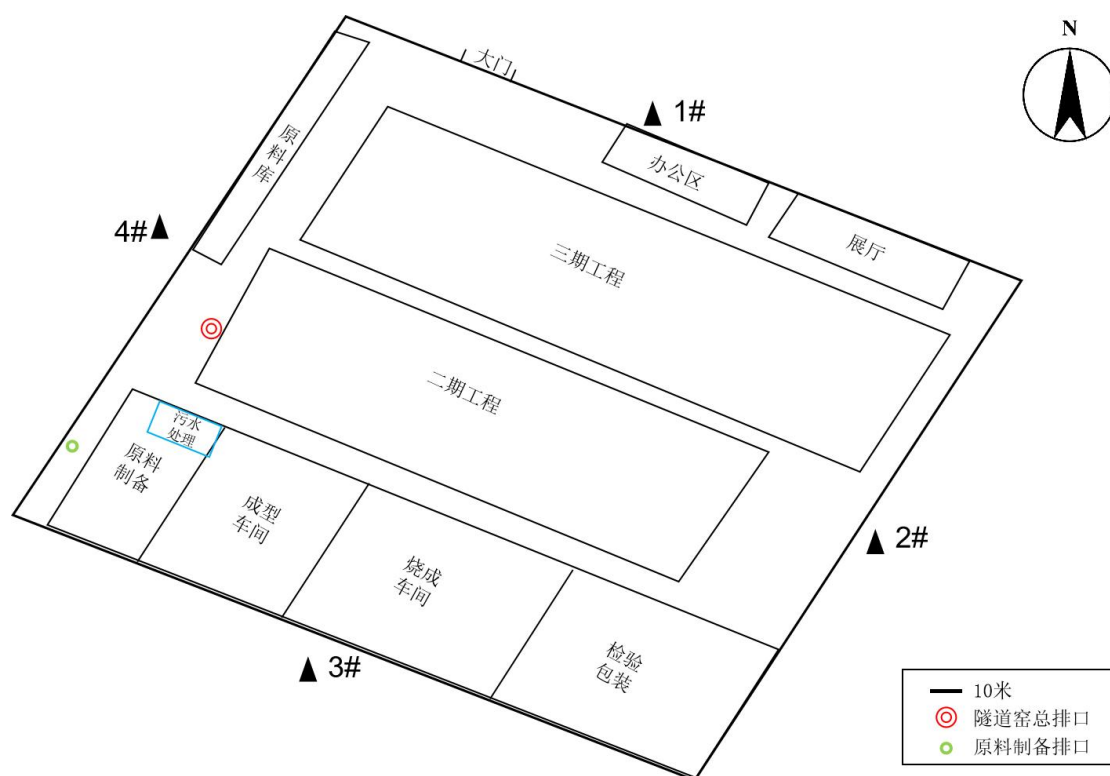
图 3-8 厂界噪声监测点位示意图
