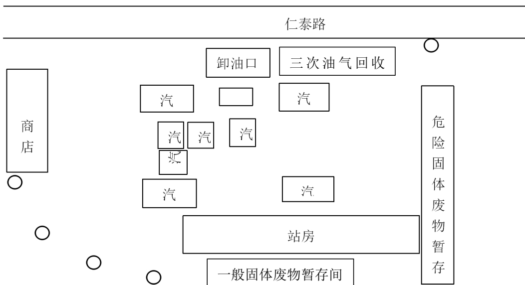
图 3-2 无组织废气监测点位示意图
