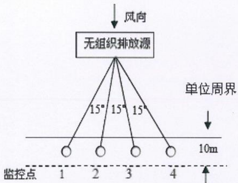
图4 无组织废气监测点位监测示意图
