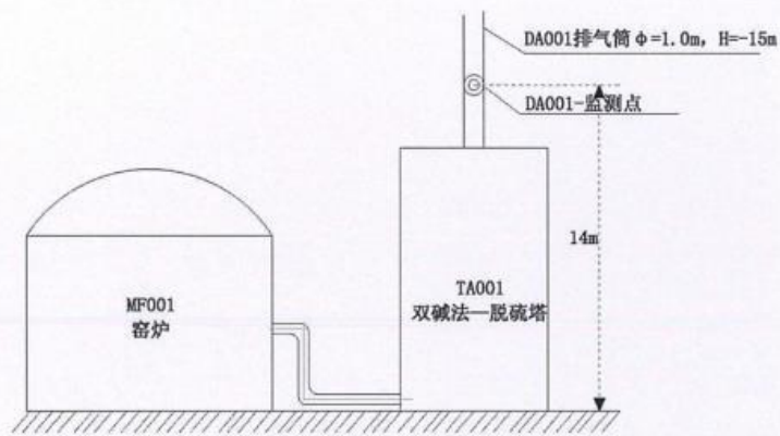
图2 隧道窑有组织监测点位监测示意图
