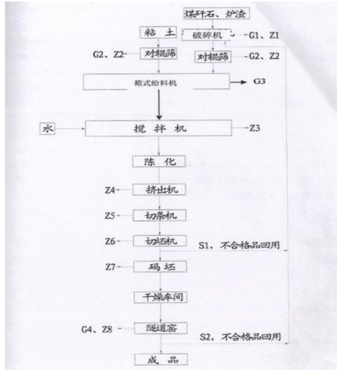
图 1 制砖生产工艺及产排污流程图
