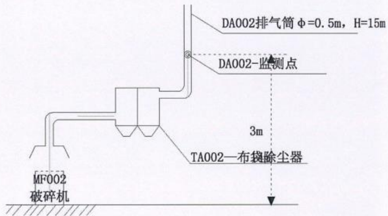
图3 筛分破碎有组织监测点位监测示意图
