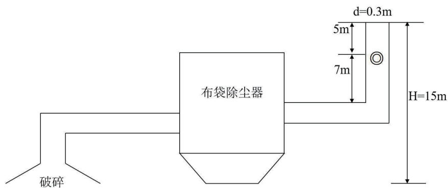
图 3-1 1#原料制备废气排放口监测点位示意图
