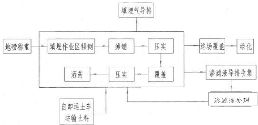
图 1-1 工艺流程图
