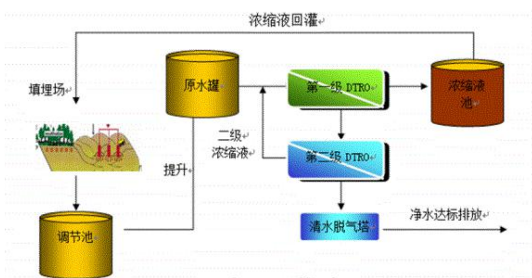
图 1-2 渗滤液处理工艺流程图
